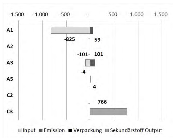
Abb.1: Holzhärente CO 2 -Produktsystemein- und -ausgänge. Die inverse Vorzeichengebung der In- und Outputs trägt der ökobilanziellen CO 2 -Flussbetrachtung aus Sicht der Atmosphäre Rechnung.
